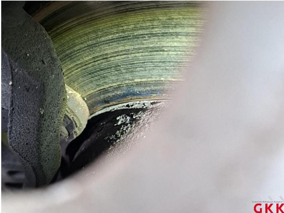
Bild 41. Bremsbeläge, vorne, Untermaß, ersetzen
