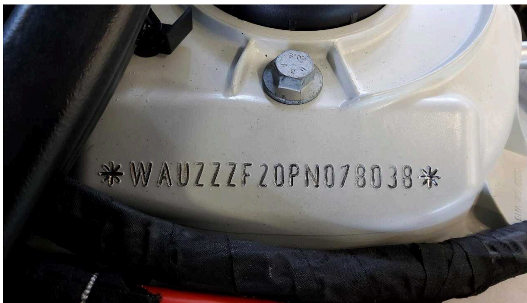
Bild 11: VIN, Fahrgestellnummer
