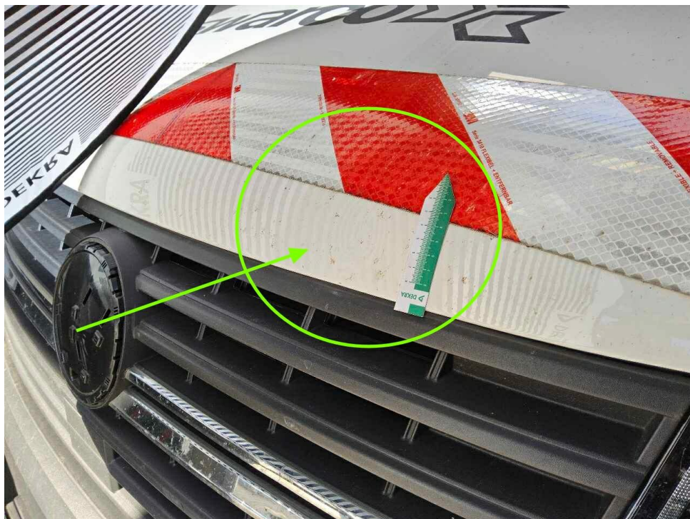
Bild 18 : Frontschaden, Stoßfänger vorne, Kühlergrill, Motorhaube
