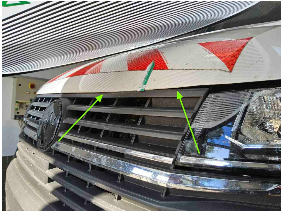
Bild 19 : Frontschaden, Stoßfänger vorne, Kühlergrill, Motorhaube
