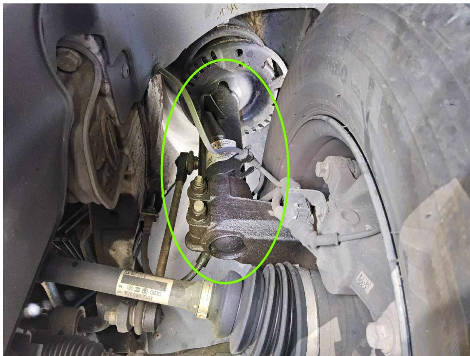
Bild 38 : Stoßdämpfer vorne links undicht
