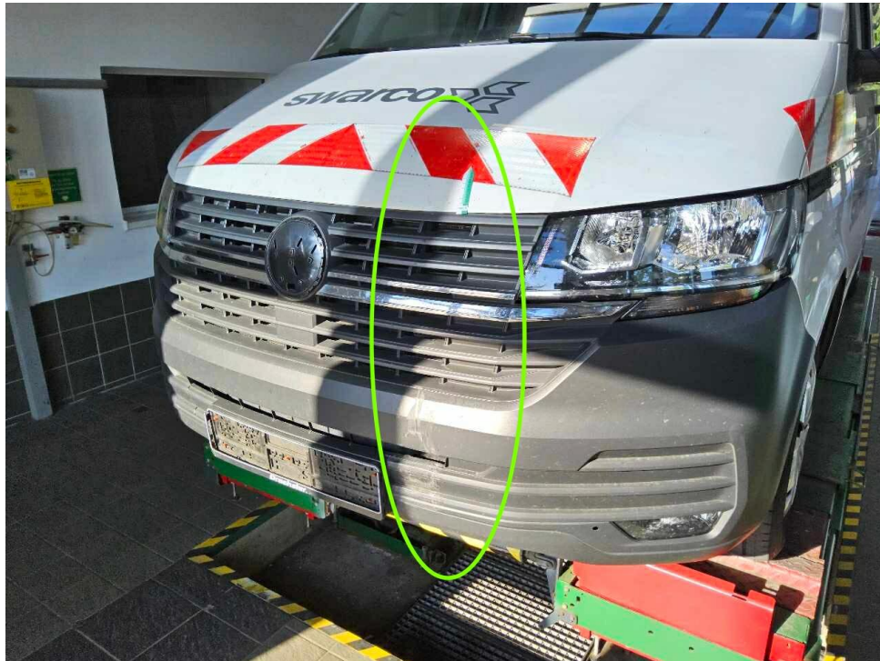
Bild 17 : Frontschaden, Stoßfänger vorne, Kühlergrill, Motorhaube
