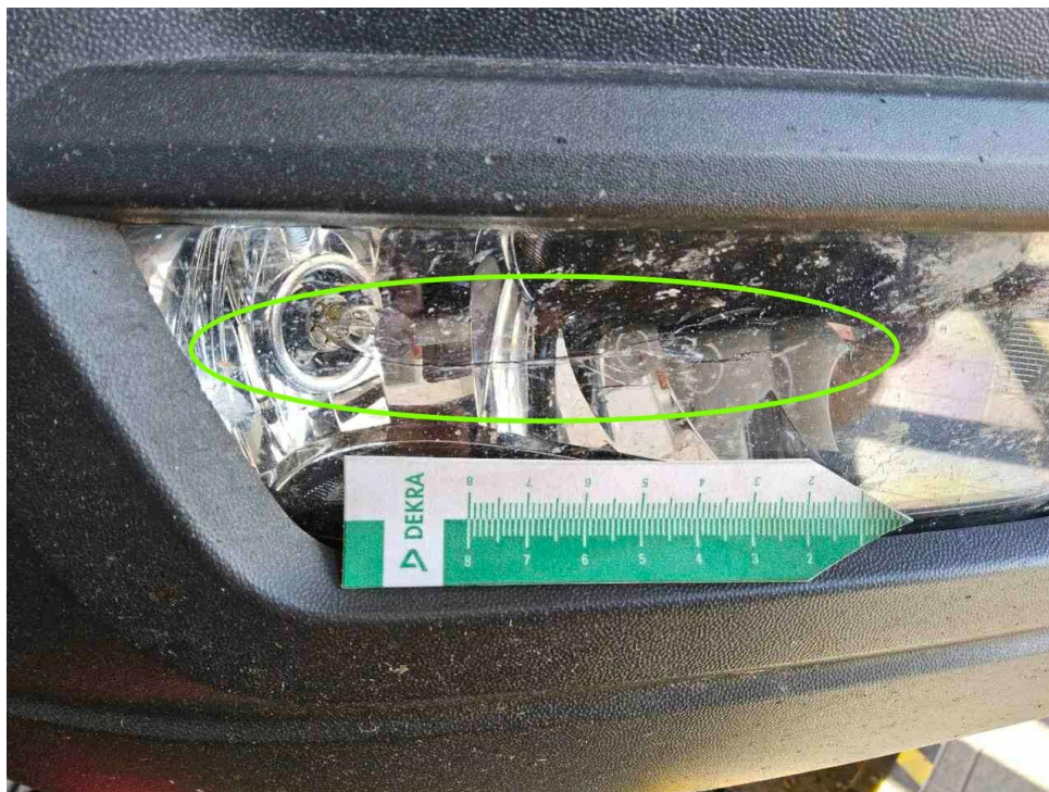
Bild 35 : Nebelscheinwerfer vorne rechts gerissen
