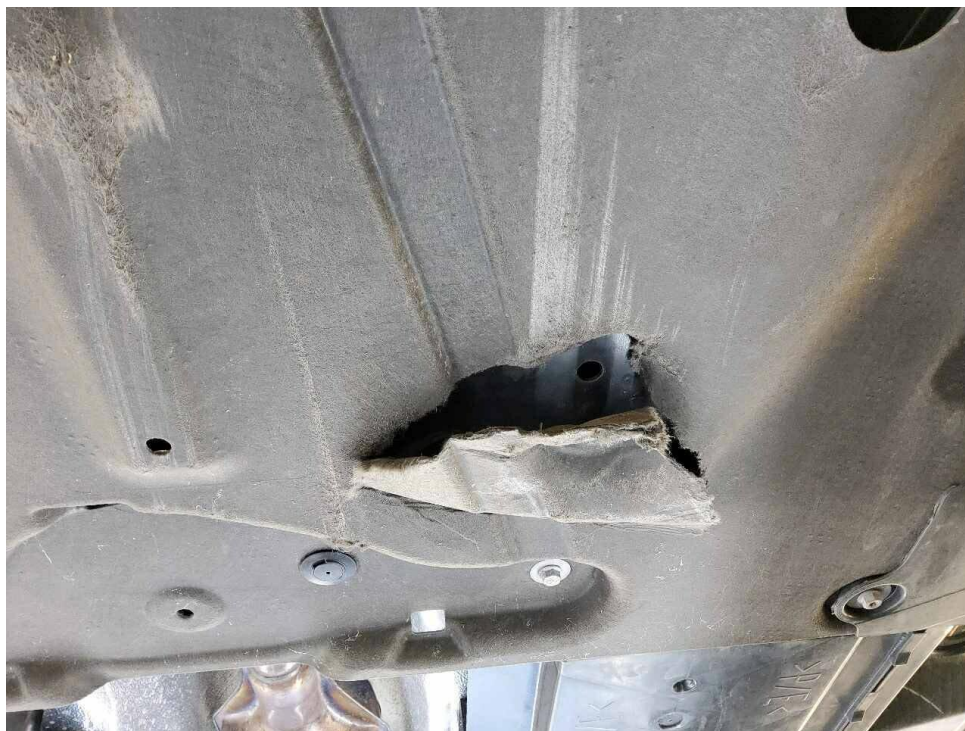
Bild 8 : Motorunterschut eingerissen
