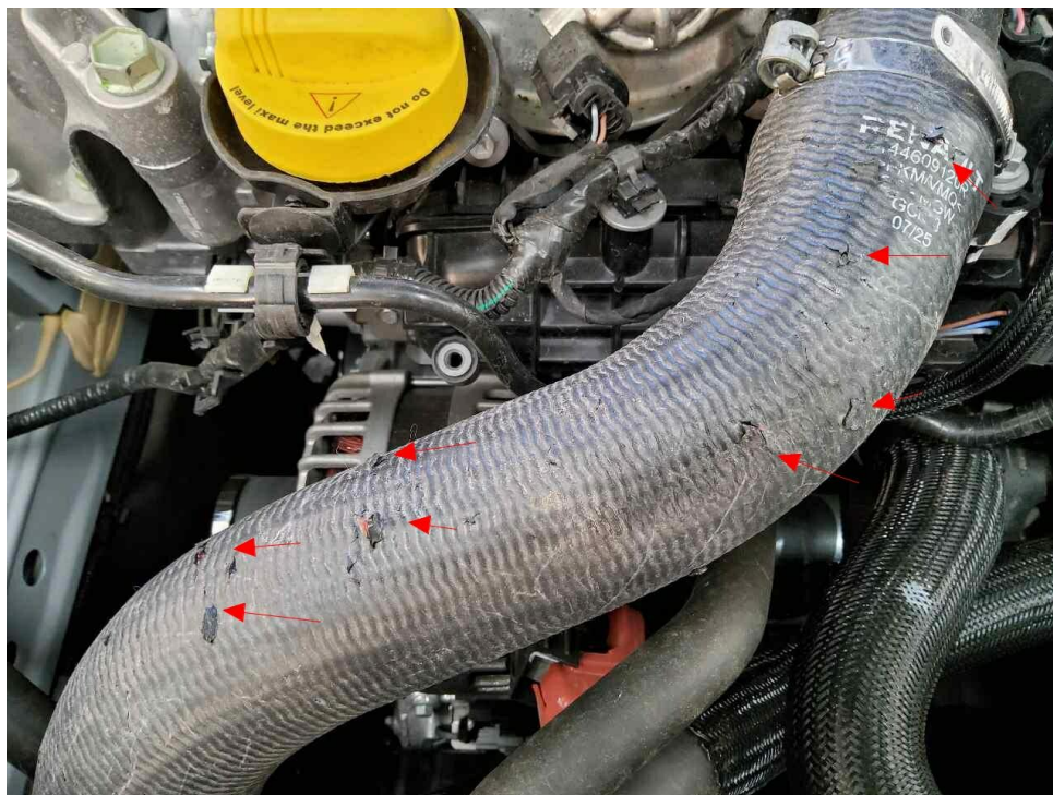
Bild 7 : Druckschlauch Ladeluftkühler Marderschaden
