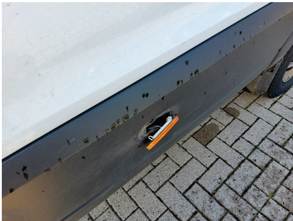
Bild 14 : Beleuchtung, Seitenmarkierungsleuchten hinten rechts+links gebrochen
