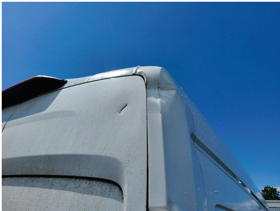
Bild 9 : Eckbeplankung rechts, eingedrückt/deformiert
