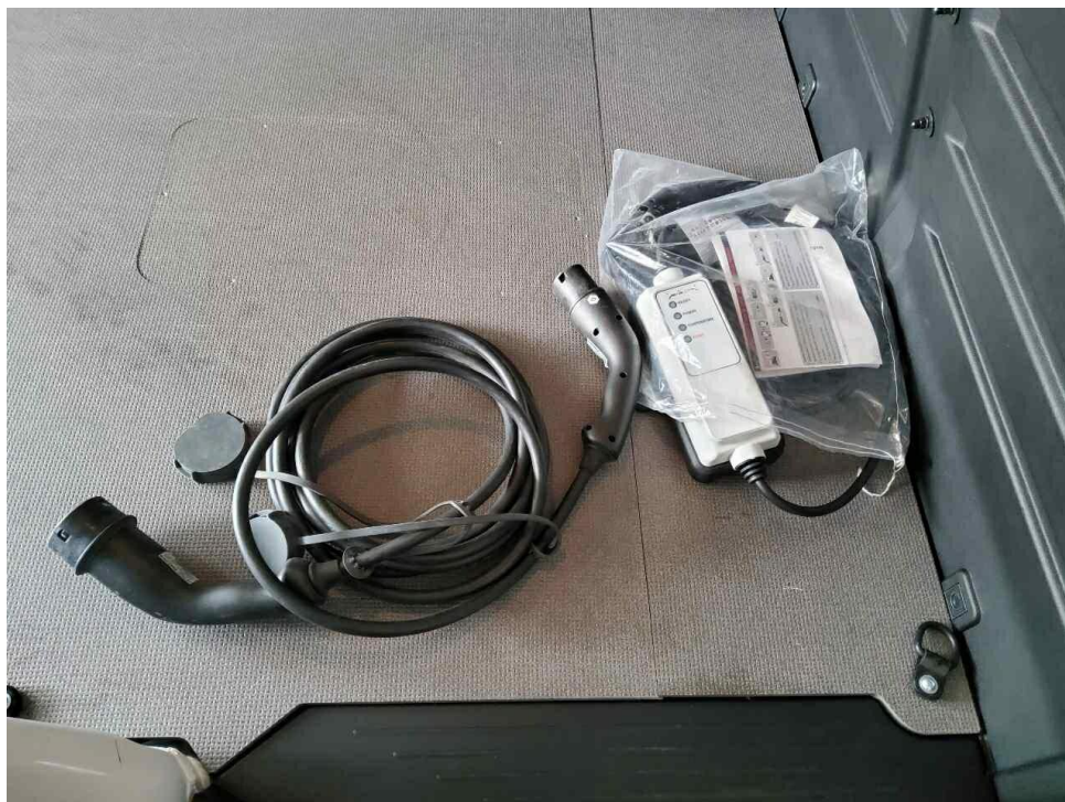
Bild 10 : Ladekabel
