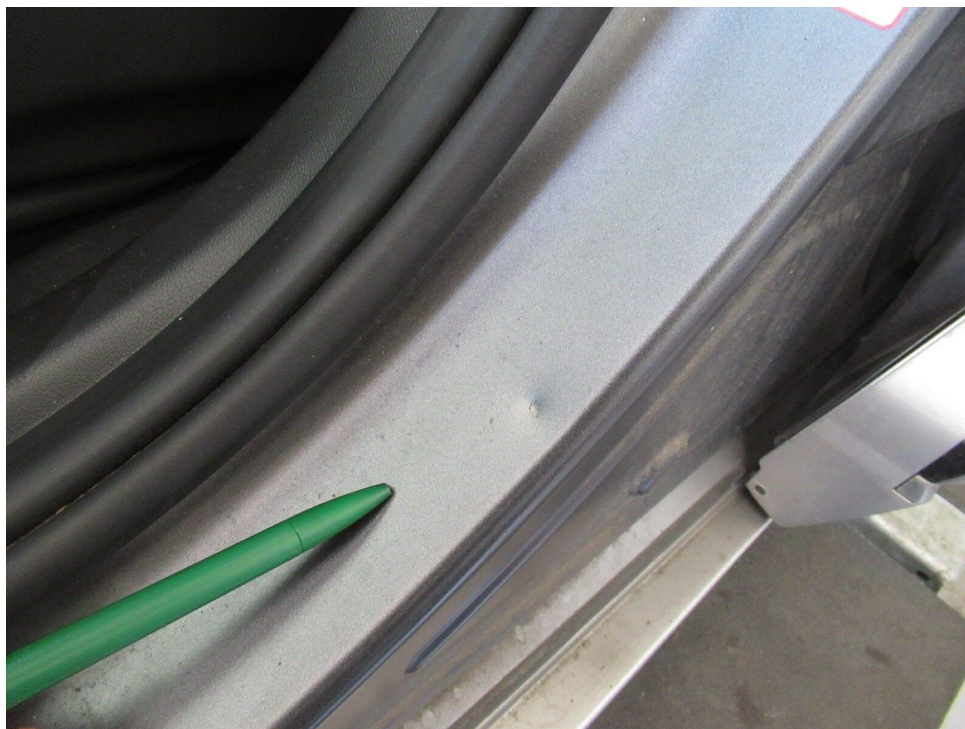
Bild 11 : Tür vorne links Einstieg, eingedellt, instandsetzen und lackieren mit Lackaufbau
