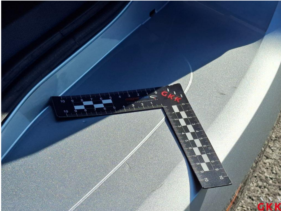
Bild 25. Stoßfänger hinten, Verkleidung -lackiert-, beschädigt, instand setzen - lackieren
