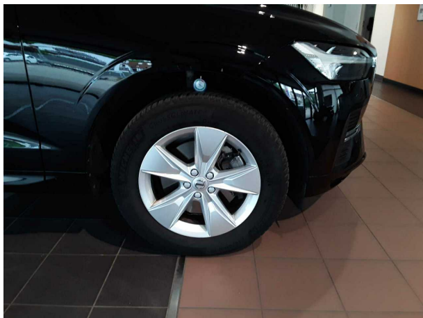
Beschädigung #1: Rad/Reifen: Reifen vorn - verschlissen - erneuern
