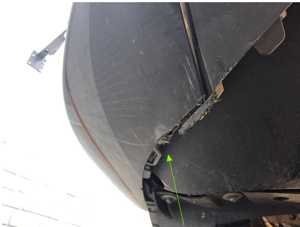
Bild 17 : Frontspoiler, gerissen, instandsetzen und lackieren mit Lackaufbau
