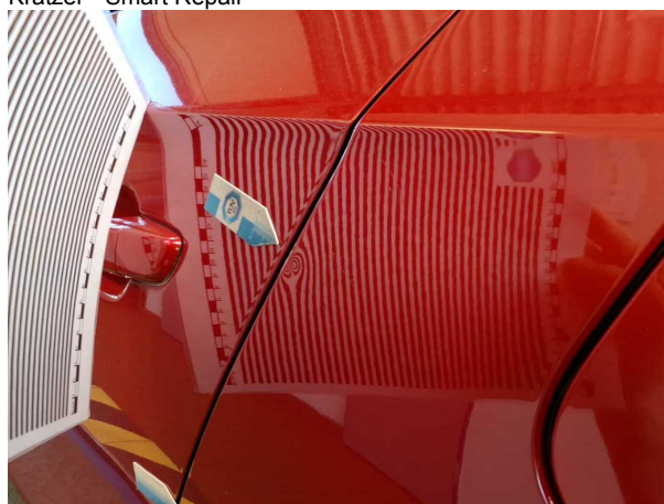
Beschädigung #5: Seitenwand links: Seitenwand - Delle / Lackschaden - Smart Repair
