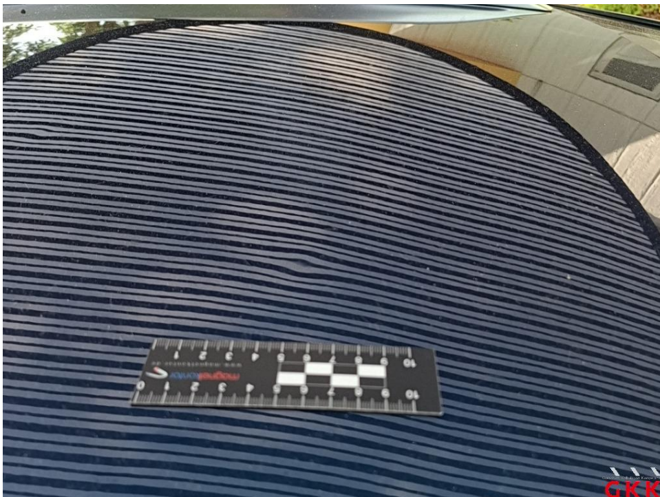
Bild 36. Dach, 4 bis 10 Dellen / Bauteil, kalt drücken
