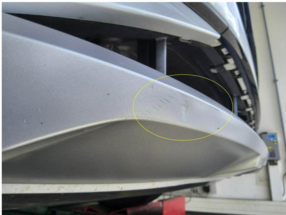
Bild 14 : Frontspoilerlippe deformiert
