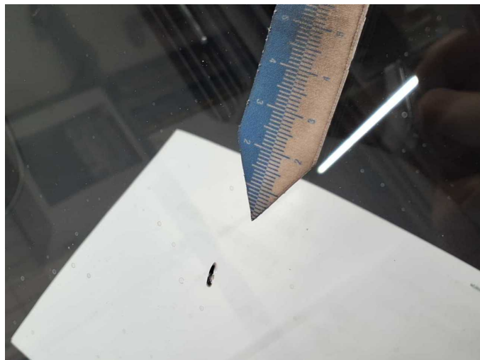
Damage 23: Vehicle glazing: Windscreen (Im Sichtbereich) - Stone chips - Replace
