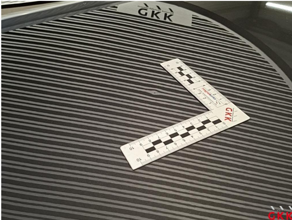
Bild 17 Dach, beschädigt, kalt drücken
