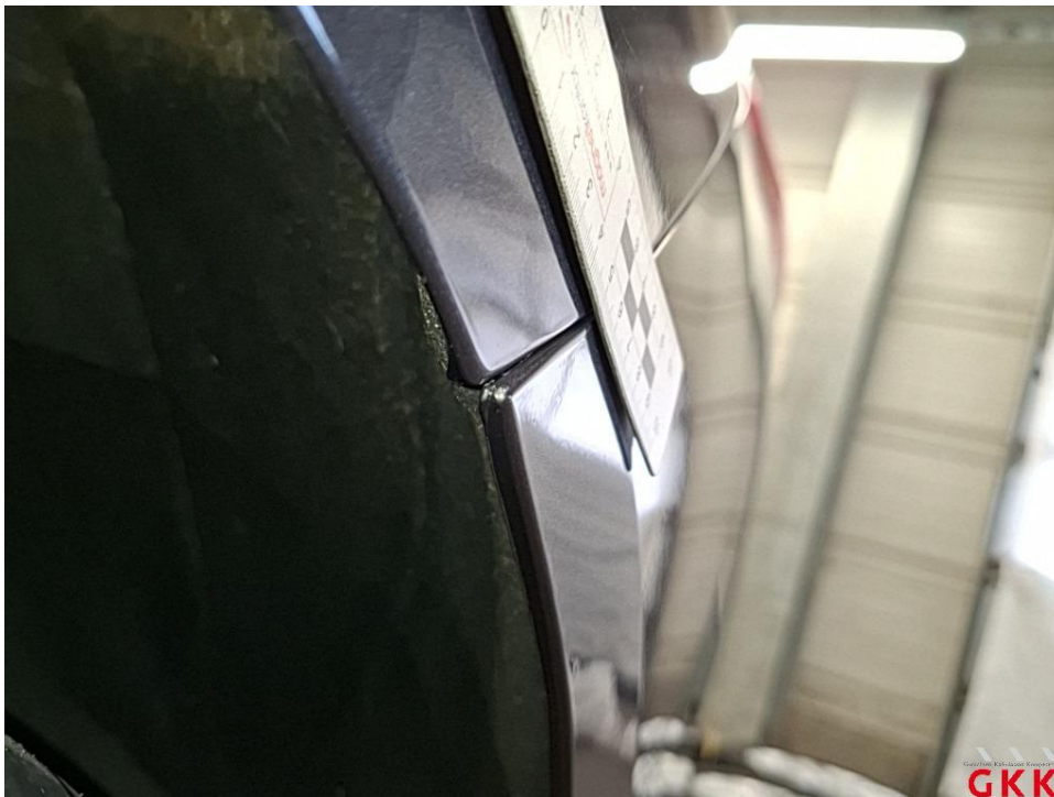
Bild 24 Stoßfänger hinten, Verkleidung -lackiert-, Spaltmaß fehlerhaft, instand setzen
