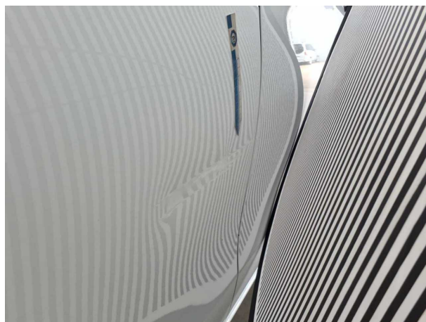
Beschädigung #20: Seitenwand rechts: Seitenwand - verformt - instandsetzen/lackieren (S2)
