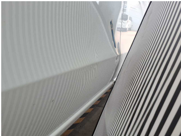
Beschädigung #18: Schiebetür rechts: Schiebetür - verformt - instandsetzen/lackieren (S2)
