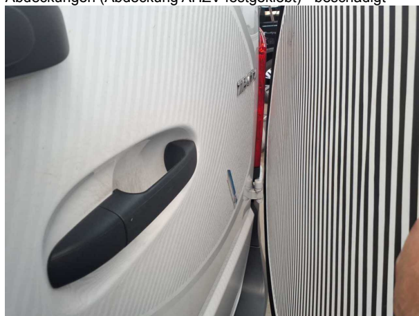
Beschädigung #4: Heckklappe/-tür: Hecktür rechts - Delle(n) - Smart Repair
