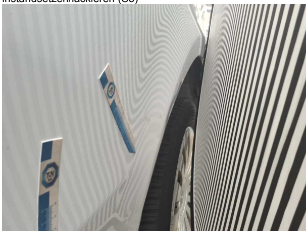
Beschädigung #19: Seitenwand links: Seitenwand - verformt - instandsetzen/lackieren (S3)
