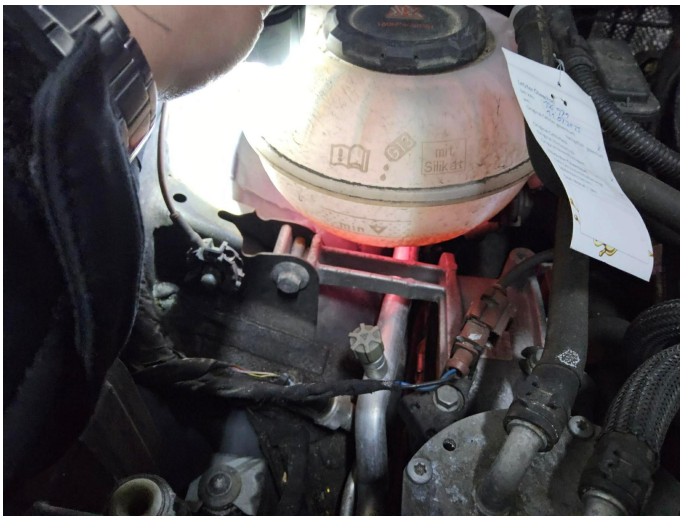
Bild 9: Technik, Flüssigkeitsstände - Kühlflüssigkeit/Frostschutz , Füllstand zu niedrig, prüfen und Befund festlegen, Schadenerweiterung möglich
