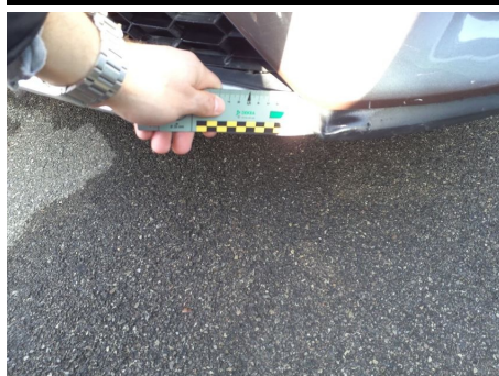
Parte inferiore paraurti / Anteriore / Rientranza
