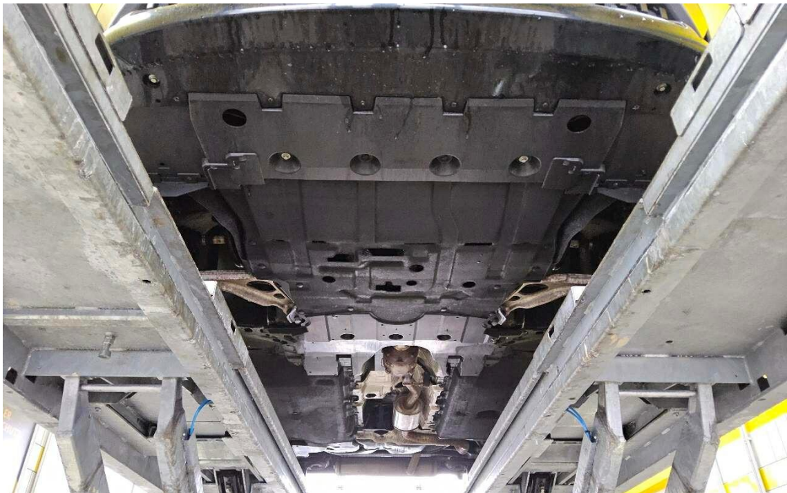
Bild 9 : Unterboden
