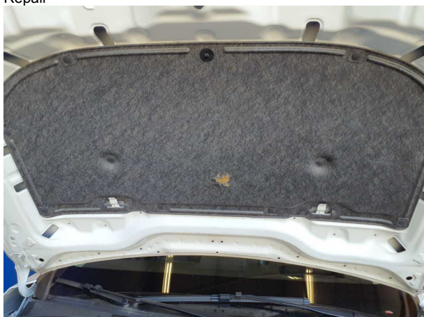
Beschädigung #2: Motorhaube: Dämmmatte - beschädigt - erneuern
