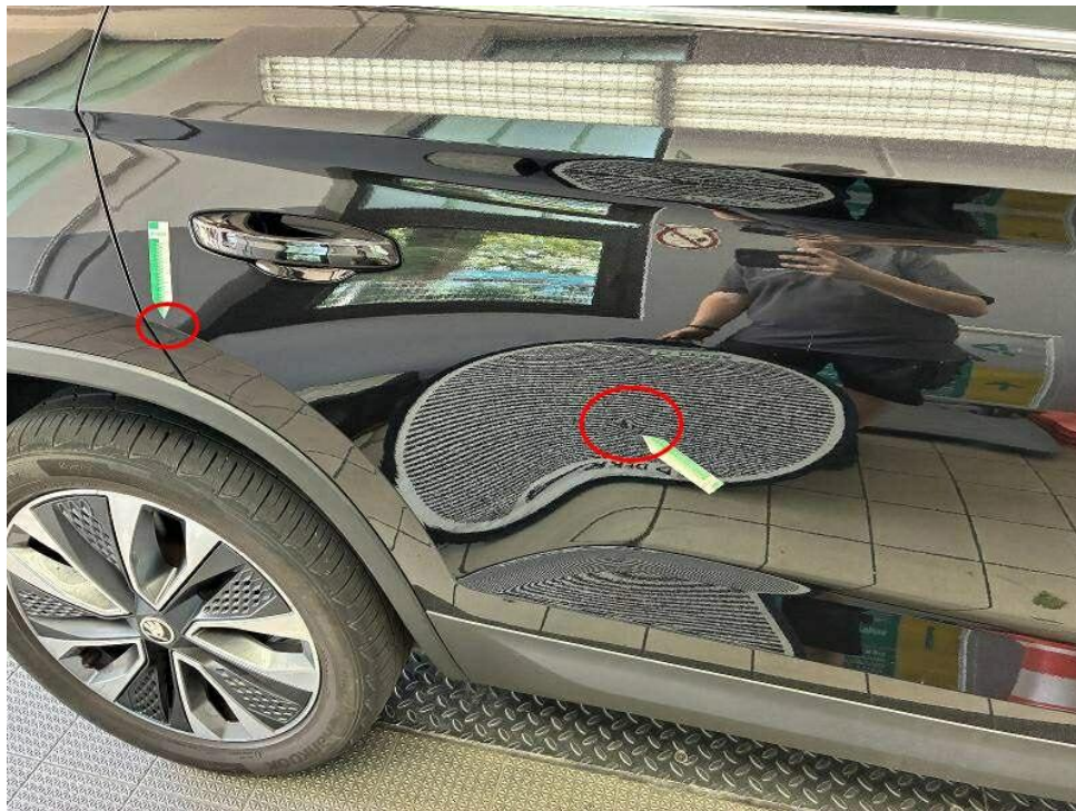
Bild 21 : Tür hinten rechts, eingedellt, instandsetzen und lackieren mit Lackaufbau
