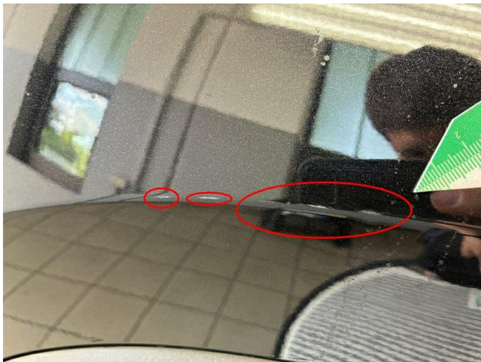
Bild 26 : Seitenteil hinten rechts, eingedellt, instandsetzen und lackieren mit Lackaufbau
