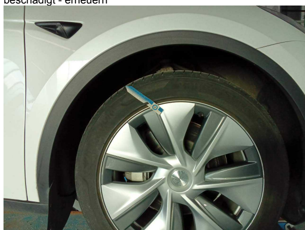
Beschädigung #5: Rad/Reifen: Reifen vorn rechts - gebrochen / gerissen - erneuern
