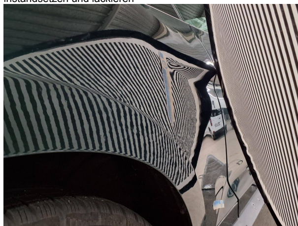
Beschädigung 7: Seitenwand rechts: Seitenwand - verformt - instandsetzen und lackieren
