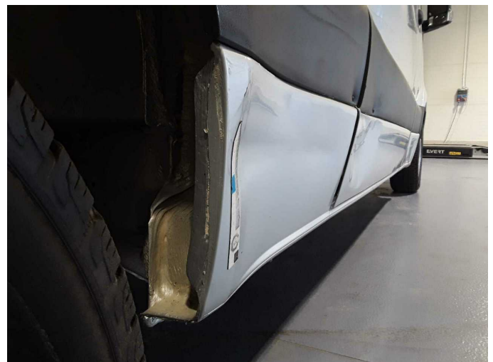
Beschädigung 14: Schweller rechts: Schweller - verformt - erneuern
