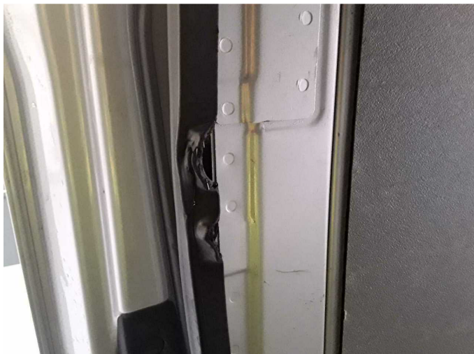
Beschädigung 28: Schiebetür rechts: Türdichtung - beschädigt - erneuern
