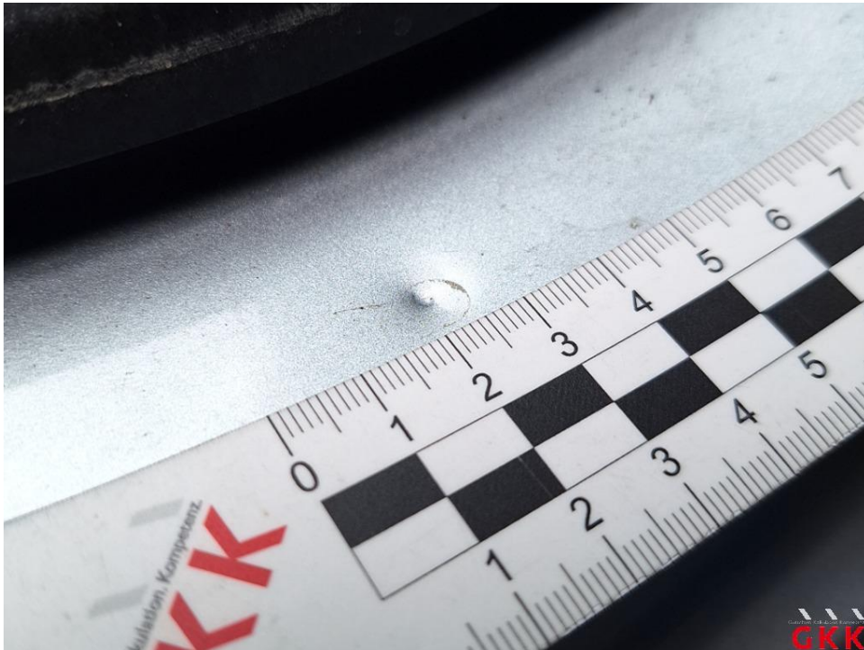
Bild 18. Tür vorne rechts, Einstieg, beschädigt, Smartrepair
