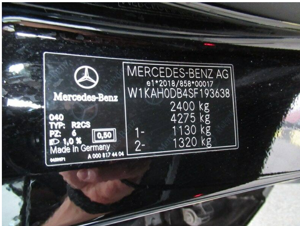
Bild 14 : Typschild
