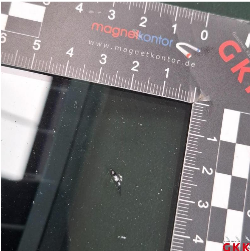
Bild 14. Frontscheibe, mit Regensensor und Frontkamera, Steinschlag mit Rissbildung, ersetzen
