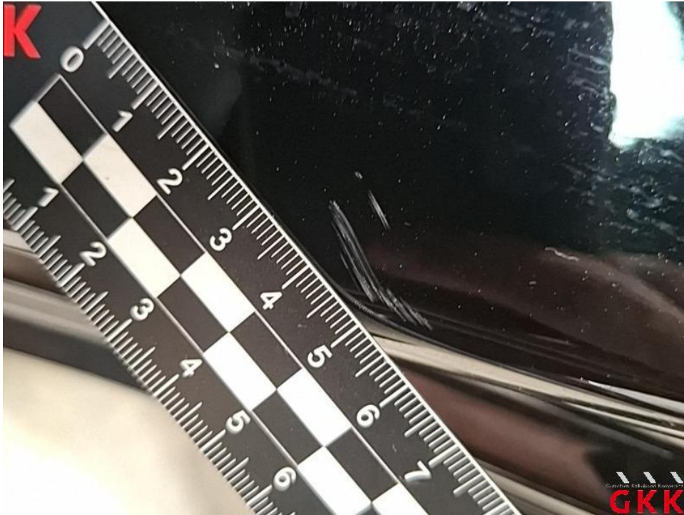
Bild 29. Tür hinten links, Einstieg, beschädigt, instand setzen - lackieren
