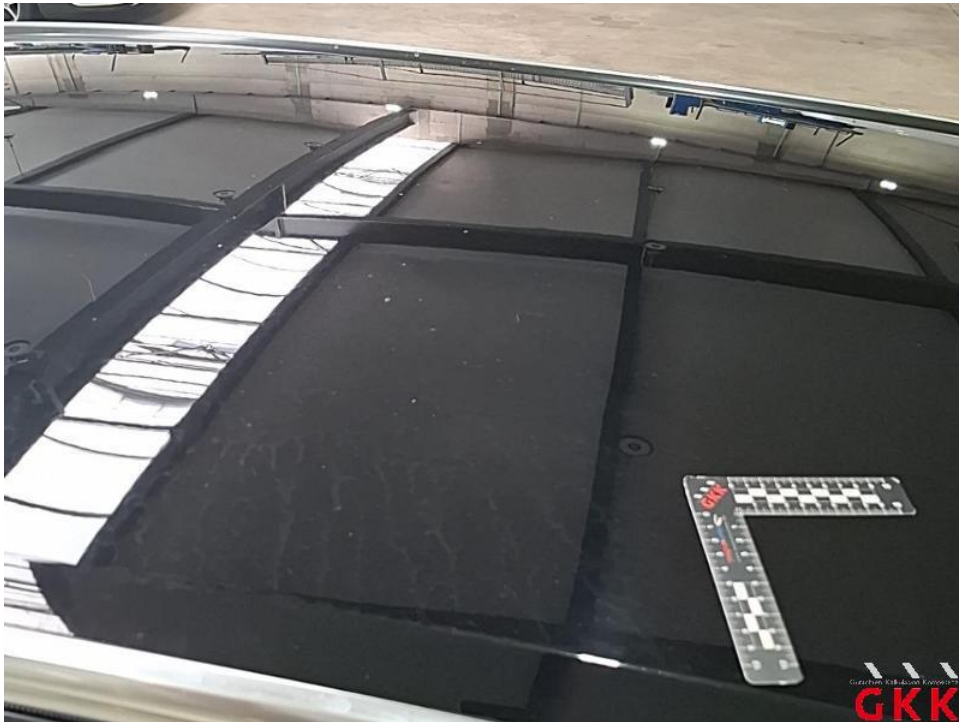
Bild 24. Dach, 4 bis 10 Dellen / Bauteil, kalt drücken
