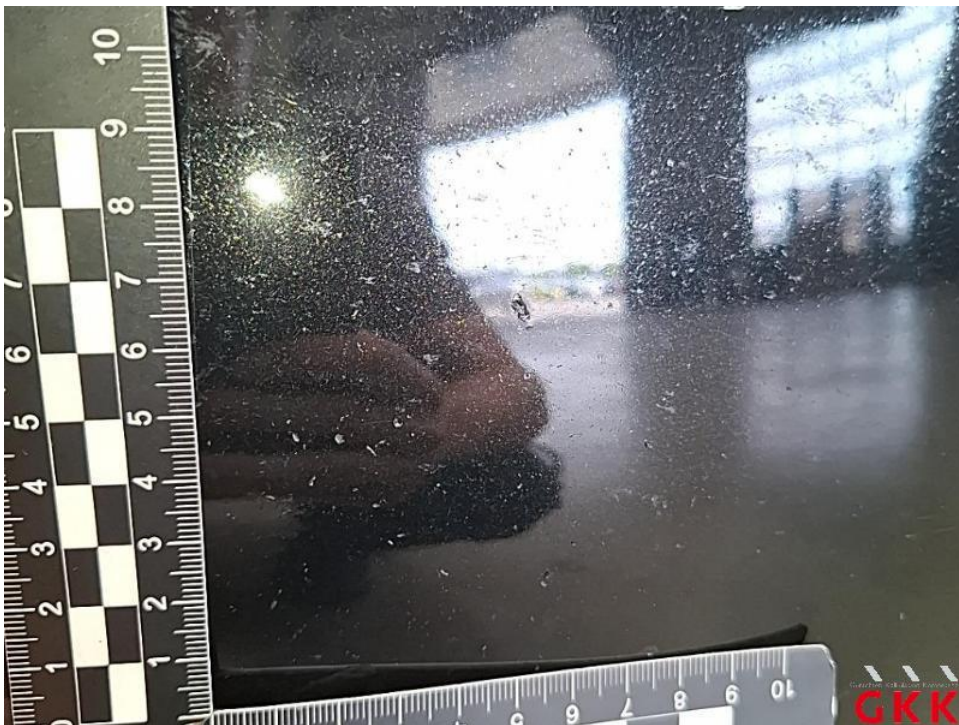
Bild 20. Stoßfänger vorne, Verkleidung -lackiert-, Steinschlag und Kratzer, lackieren
