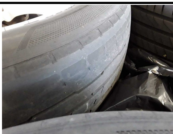
Beschädigung #6: 2.Radsatz: 2 Reifen (außen abgefahren) - verschlissen - erneuern
