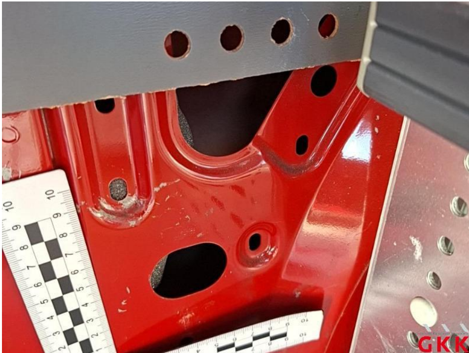
Bild 32. Seitenwand links, innen, verkratzt, Spotlackieren
