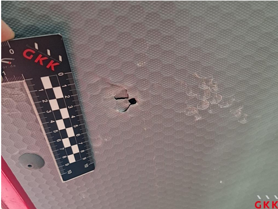
Bild 21. Heckklappe, Innenverkleidung, beschädigt, ersetzen
