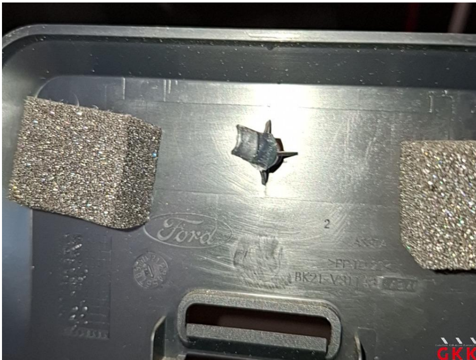
Bild 16 Innenraumverkleidung, beschädigt, ersetzen
