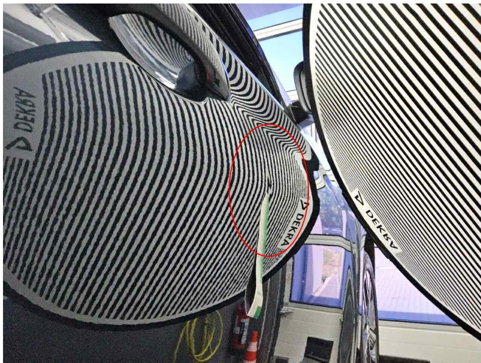
Bild 13 : Türe vorne rechts eingedellt
