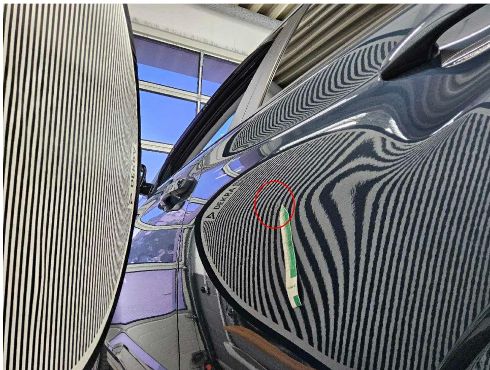
Bild 11 : Türe hinten links eingedellt
