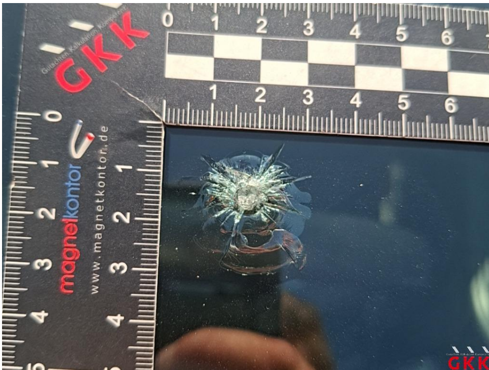
Bild 22. Frontscheibe, mit Regensensor und Frontkamera, Steinschlag im Sichtfeld, ersetzen
