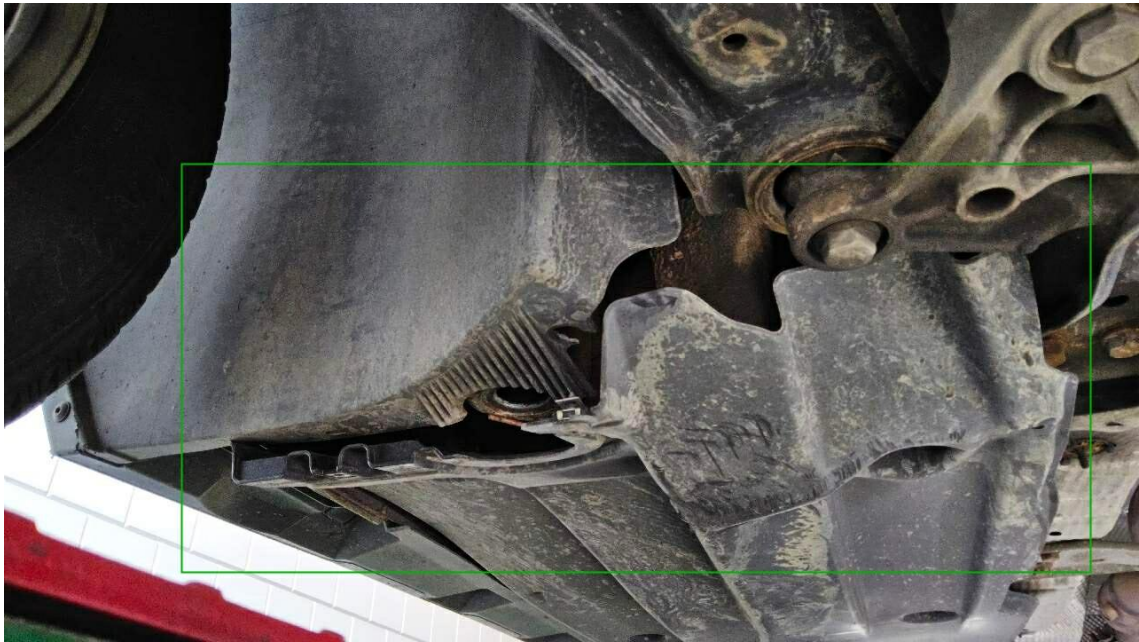
Bild 47 : Unterbodenverkleidung mitte rechts und Radhausschale vorne rechts, gebrochen
