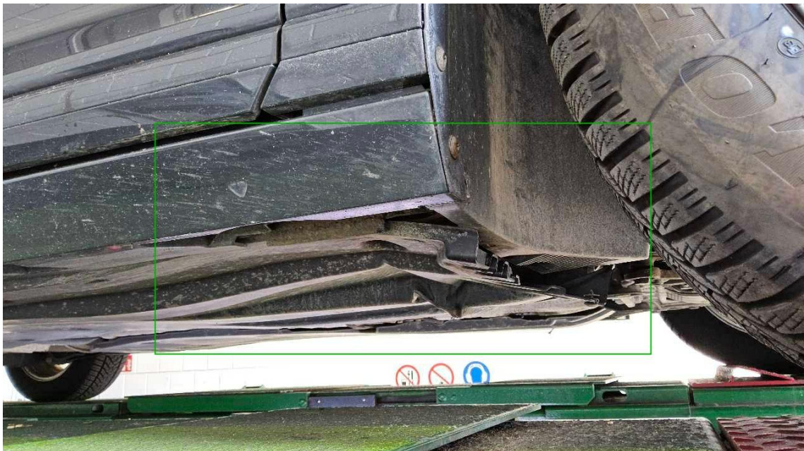
Bild 50 : Unterbodenverkleidung mitte rechts und Radhausschale vorne rechts, gebrochen
