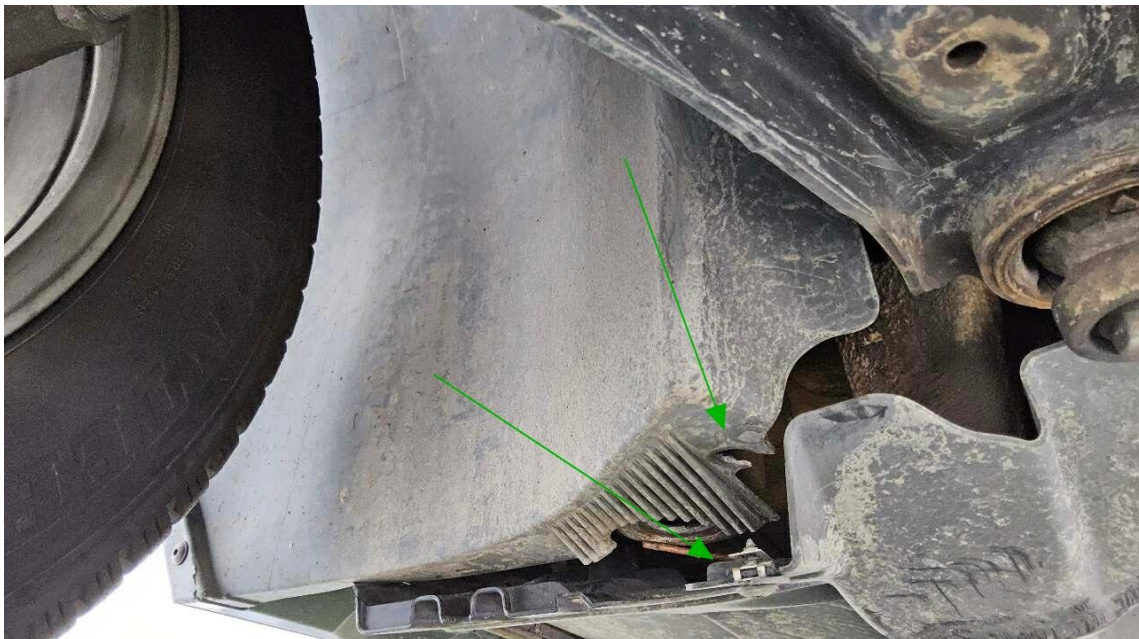
Bild 48 : Unterbodenverkleidung mitte rechts und Radhausschale vorne rechts, gebrochen
