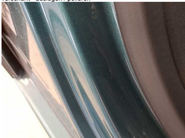
Beschädigung #2: Schweller rechts: Einstieg - Delle(n) - sanft instandsetzen
