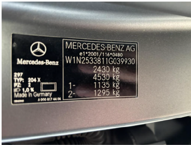
Typenschild/VIN
