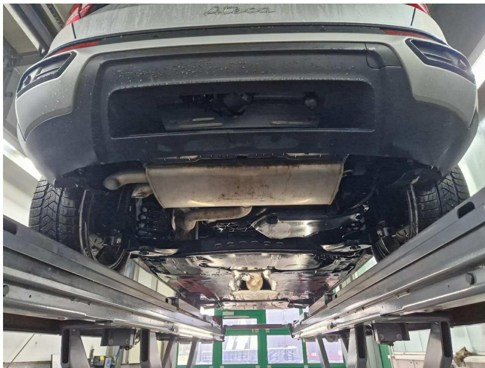
Bild 26 : Unterboden hinten
