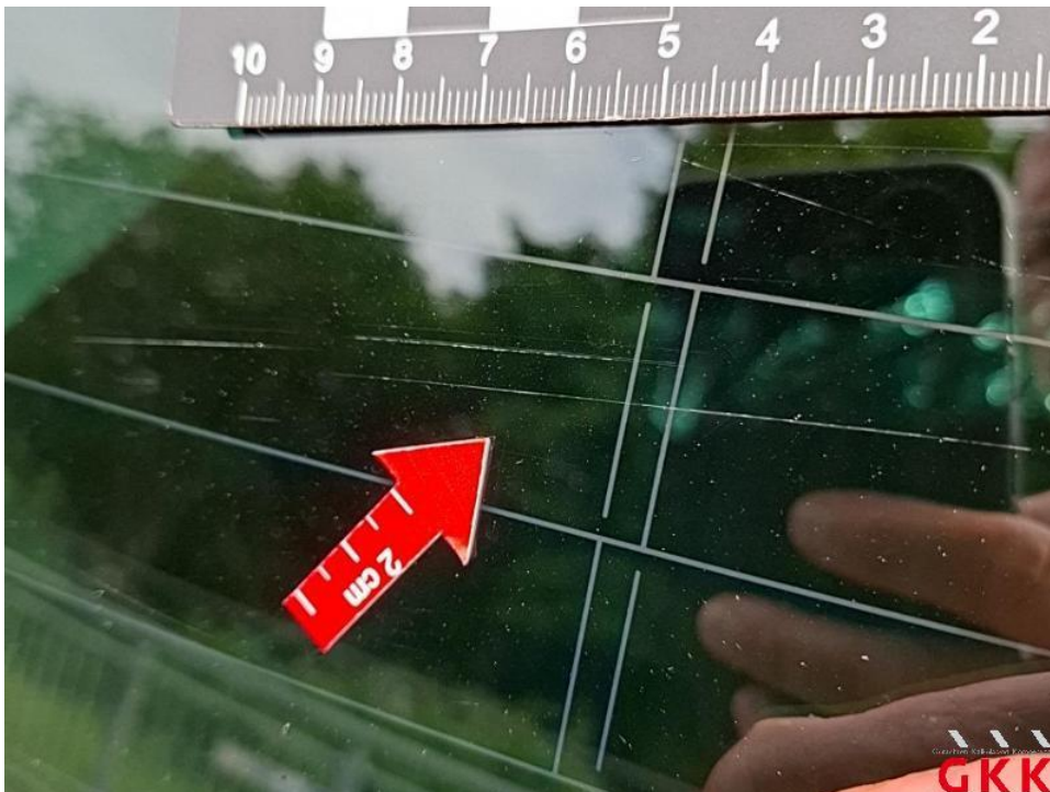
Bild 38. Heckscheibe, getönt, verkratzt, ersetzen
