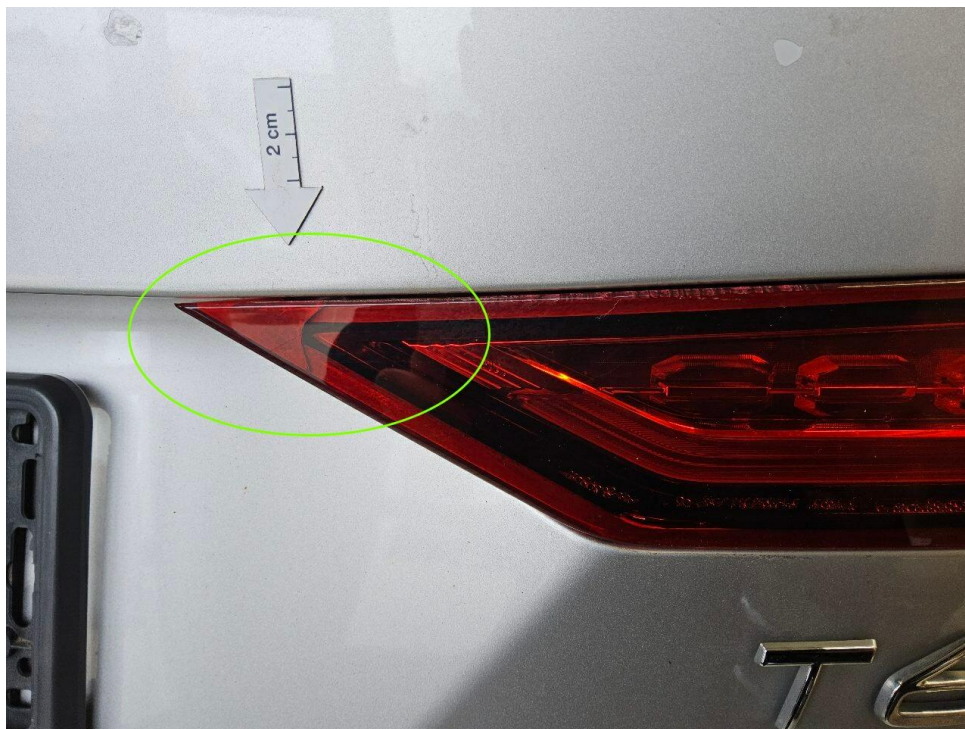
Bild 25 : Heckklappe Rücklicht, gebrochen
