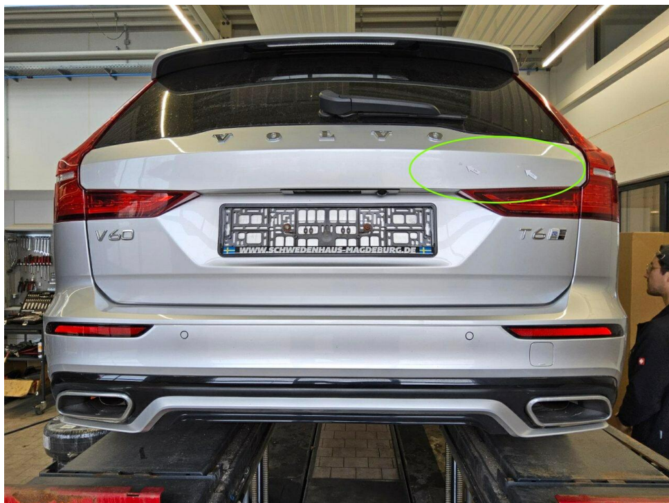
Bild 24 : Heckklappe Lackierung, zerkratzt, lackieren mit Lackaufbau
