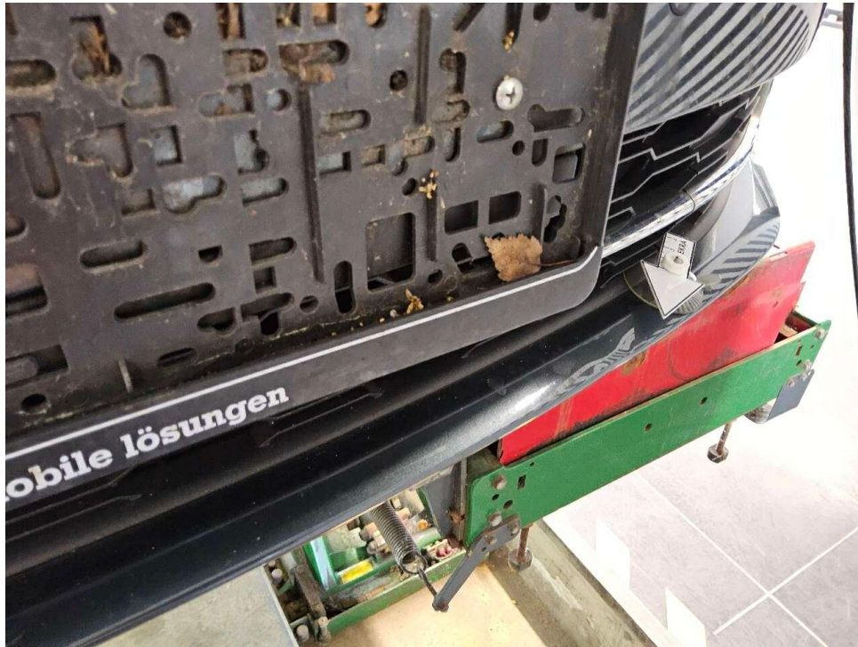
Bild 37 : Stoßfänger vorne, eingedellt, instandsetzen und lackieren mit Lackaufbau
