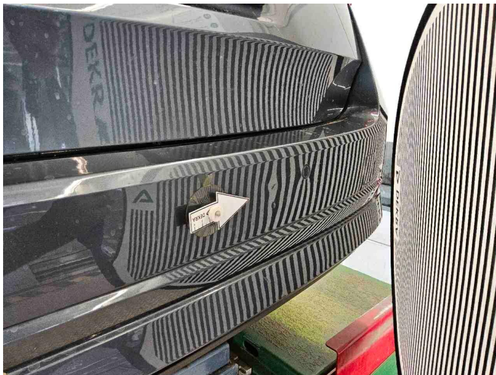
Bild 23 : Stoßfänger hinten, eingedellt, instandsetzen und lackieren mit Lackaufbau
