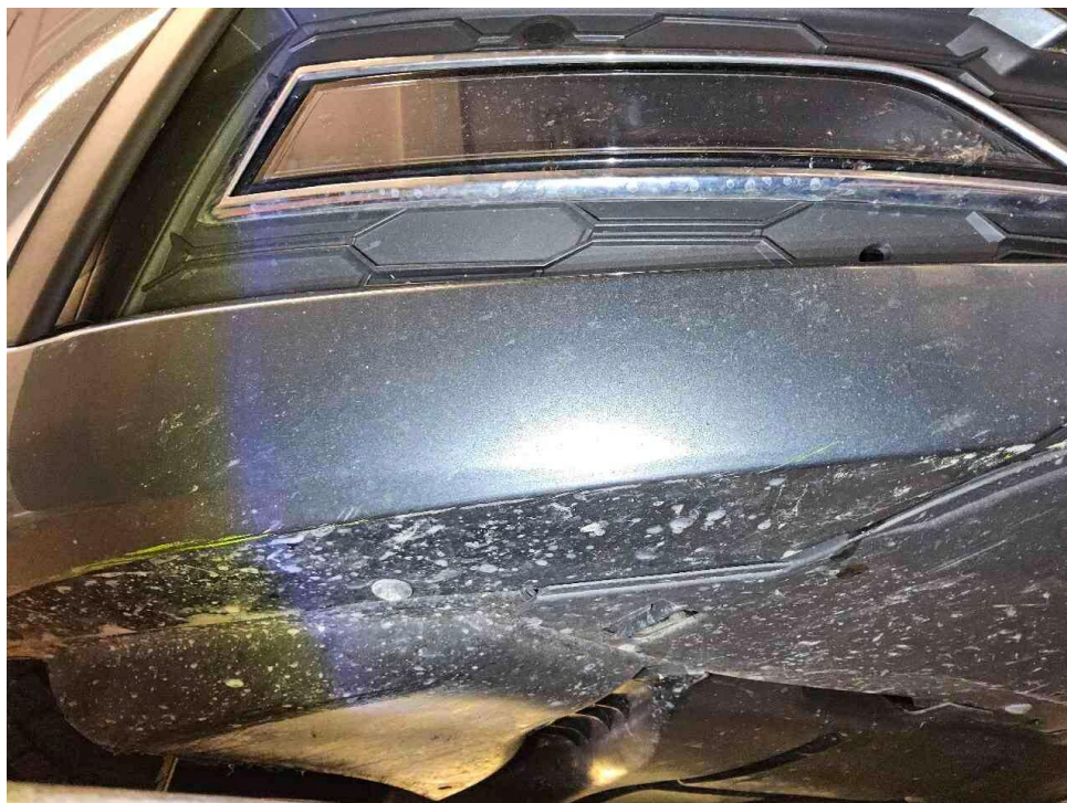
Bild 38 : Stoßfänger vorne, eingedellt, instandsetzen und lackieren mit Lackaufbau
