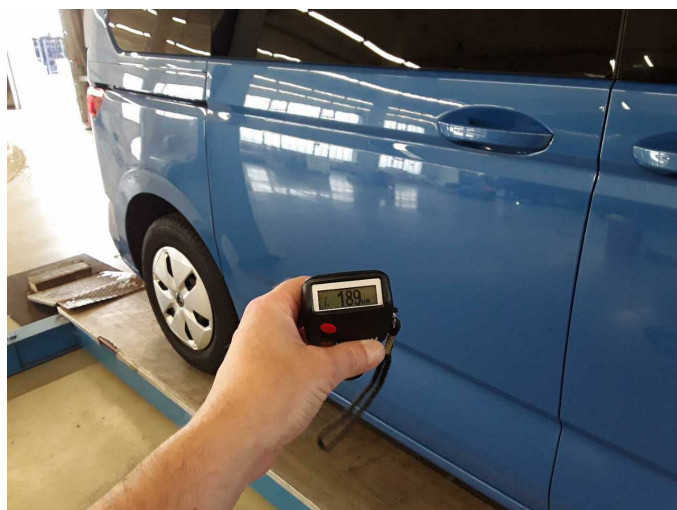
Door - rear right side: 189 \mu\text{m}
