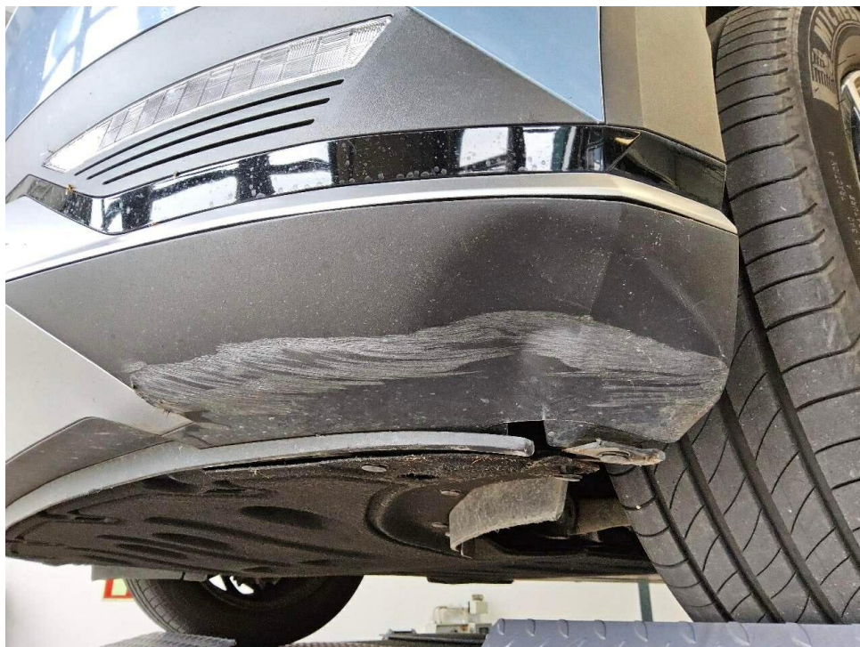
Bild 8 : Frontspoiler vorne links verformt/ destrukturiert/ verschrammt
