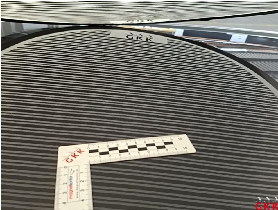
Bild 16 Dach, 4 bis 10 Dellen / Bauteil, kalt drücken
