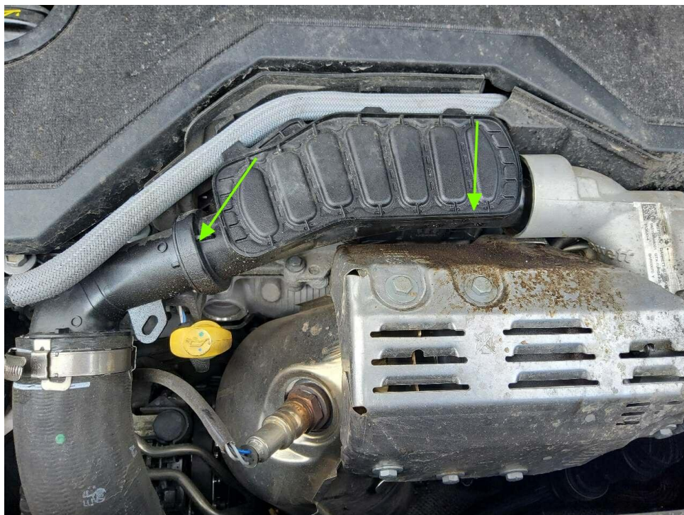
Bild 12 : Motor, undicht
