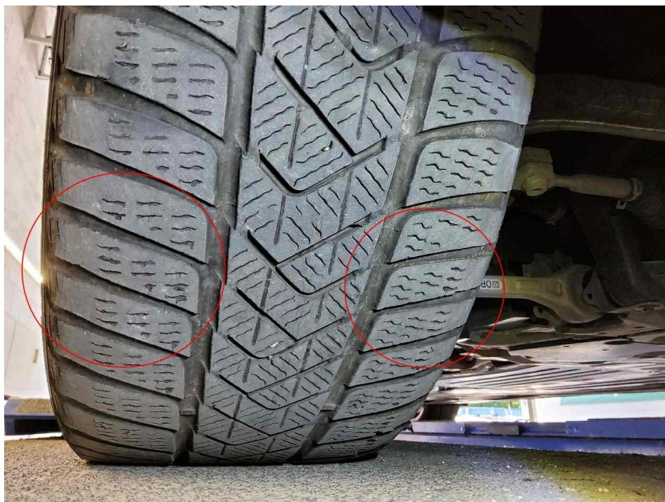
Bild 24 : Alle Winterreifen, verschlissen vorne rechts
