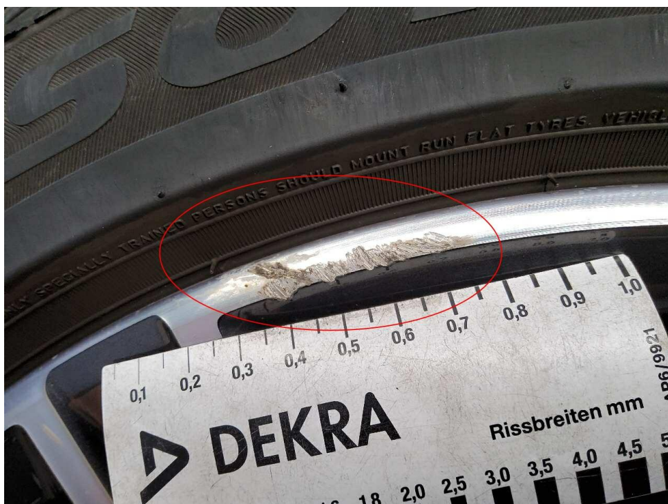
Bild 20 : LM-Felge vorne rechts (Winter), glanzgedreht, verschrammt
