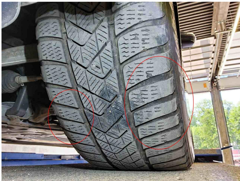
Bild 25 : Alle Winterreifen, verschlissen vorne links
