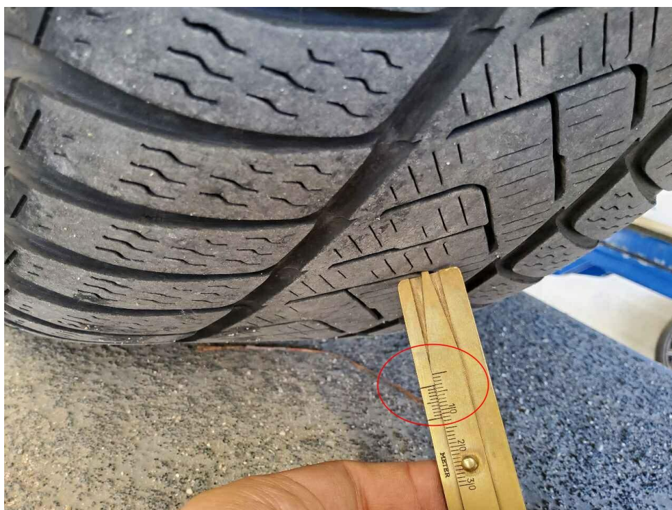
Bild 26 : Alle Winterreifen, verschlissen hinten links
