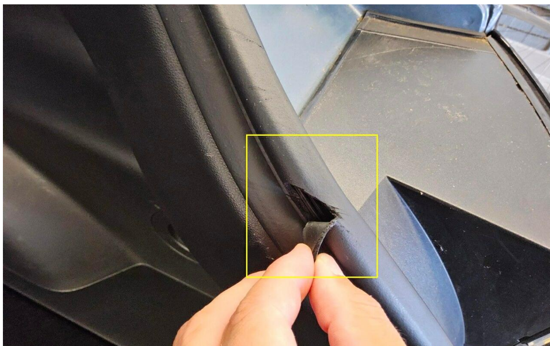
Bild 7 : Heckklappendichtung eingerissen
